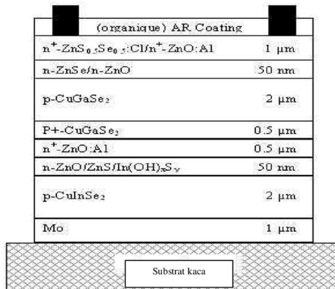
Gambar 7. Sel surya tandem basis CIS dan CGS [7]
