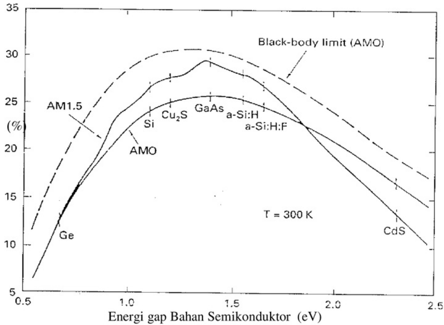
Gambar 5. Efisiensi berbagai bahan sel surya sebagai fungsi dari energi gap.
