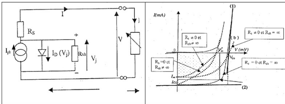
Gambar 3. (a). Skema ekivalen sebuah sel surya .
