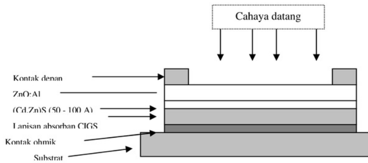
Gambar 6. Sel surya CIGS : MgF 2 /ZnO:Al/ZnS:CIGS/Mo/Substrat [10]
