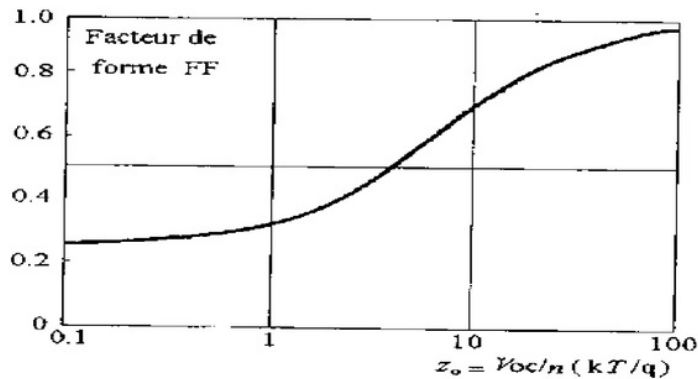
Gambar 4. Faktor bentuk FF sebagai fungsi z_o menurut [3]
