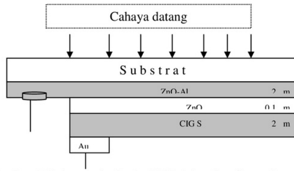
Gambar 5. Sel surya berbasis CIGS dalam konfigurasi superstrate [9]
