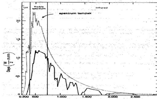
Gambar 1. Penyebaran panjang gelombang cahaya surya di atas atmosfer (garis titik-titik) dan di permukaan bumi (garis hitam)
